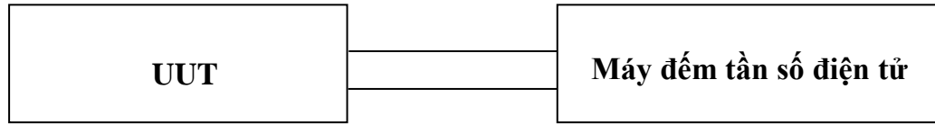
Hình 2 : Sơ đồ kiểm tra tần số thiết lập và độ ổn định tần số
